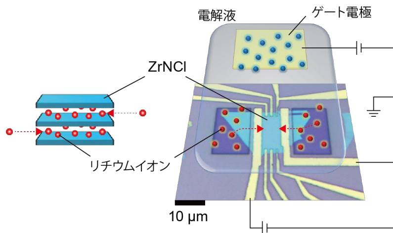
図2. ZrNCl を用いたイオンゲートデバイスの模式図。ZrNCl の層間に入るリチウムイオンの量を、ゲート電圧によって制御することができる。
